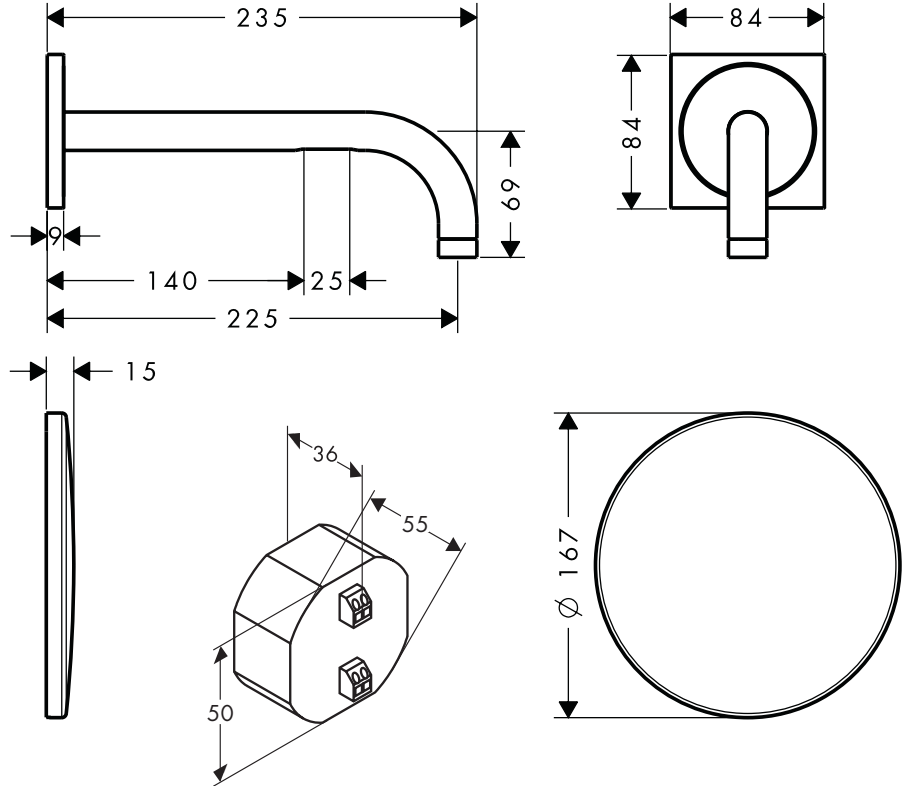
AXOR Uno 38120000
