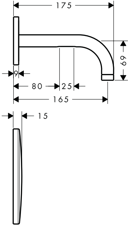
AXOR Uno 38119000
