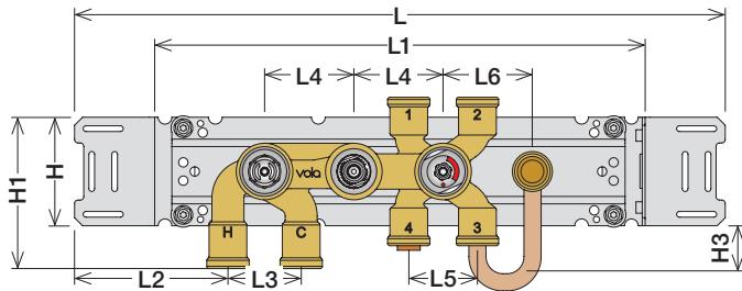
C: 5400NVA3 D: 5400FVA3
