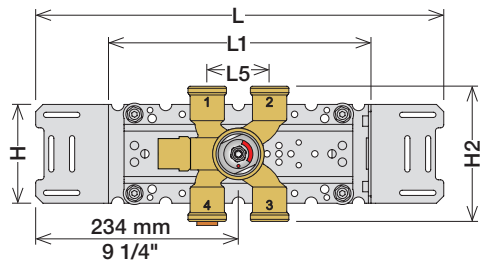
C: 5400NVA3 D: 5400FVA3
