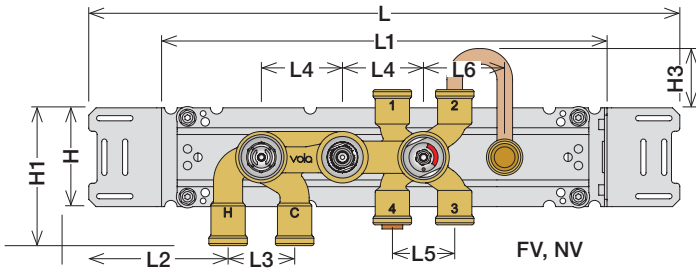
C: 5400TVA3 D: 5400RVA3
